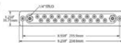
EBB2-20
