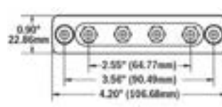
EMB4
