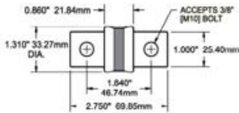
225-400 Amperes
